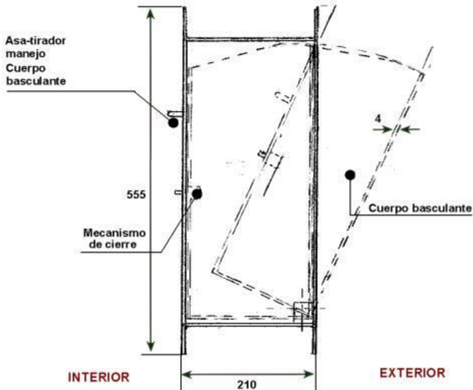
Vista perfil
