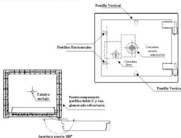
DIBUJOS VISTA FRONTAL Y PLANTA
